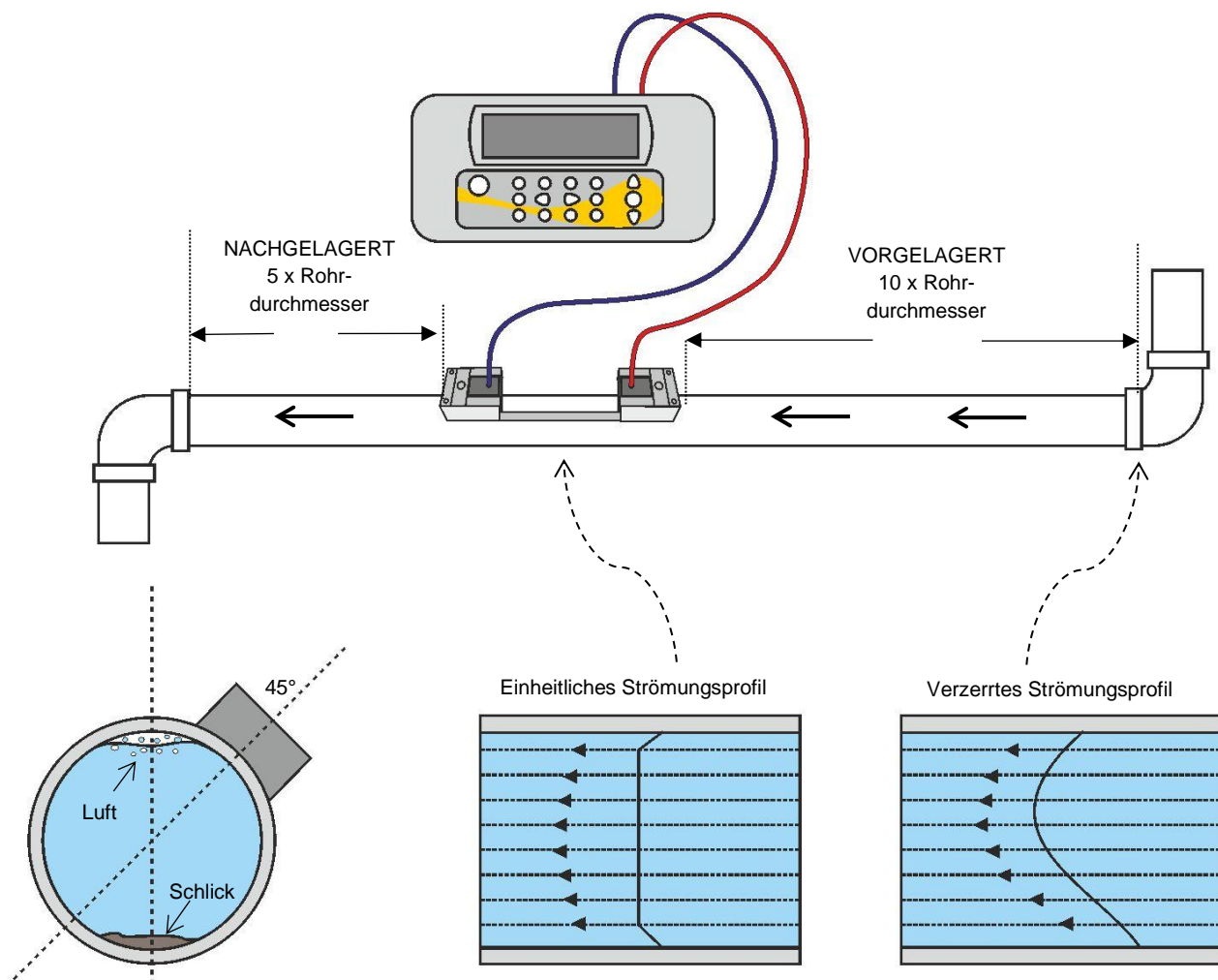
Abbildung 8 Positionierung des Geräts
