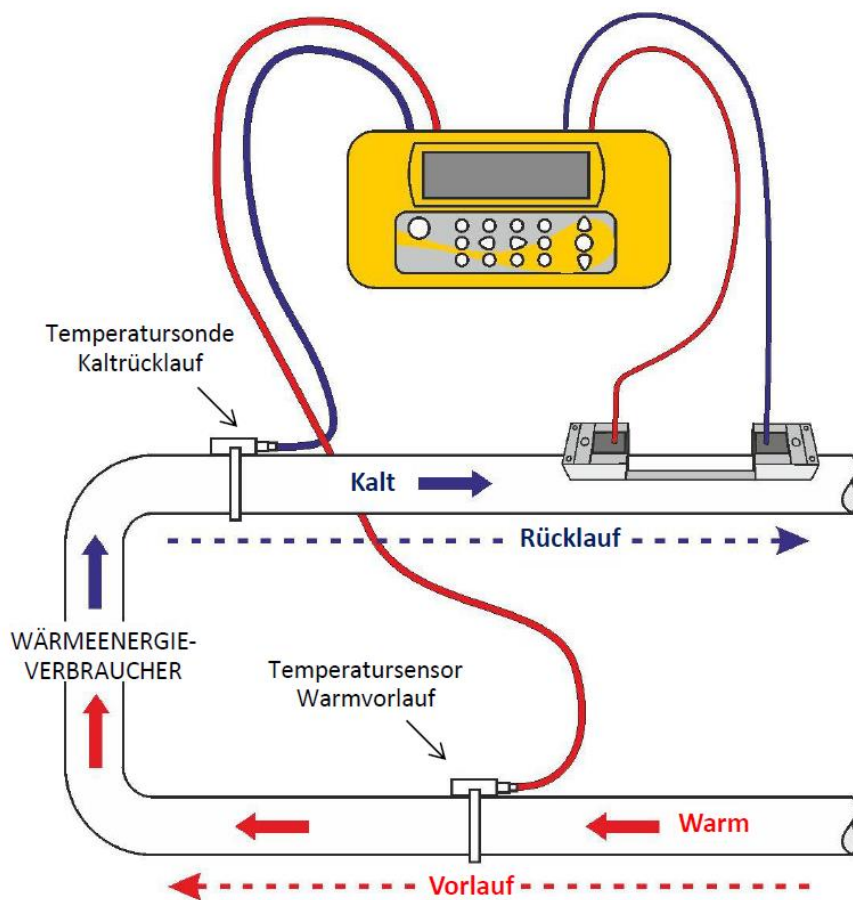
Abbildung 13 Positionierung Temperatursonde Portaflow 333 (Heizsystem)
