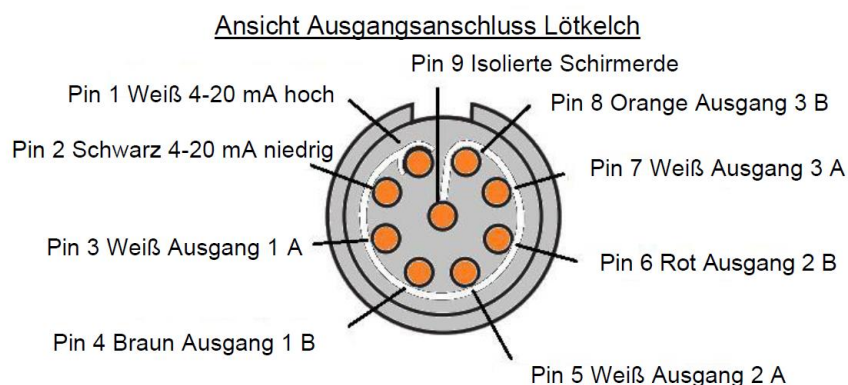
Abbildung 15 Ausgangverkabelung
