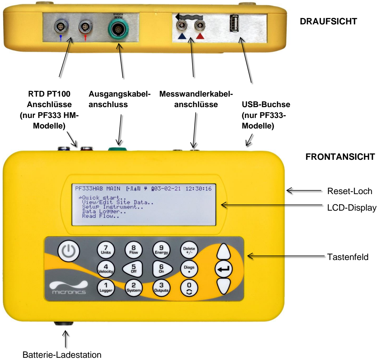
Abbildung 5 Portaflow-Einheit (Modell PF333HM abgebildet)
