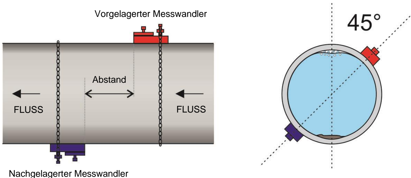
Abbildung 12 Messwandlerpositionen für den Diagonalmodus
