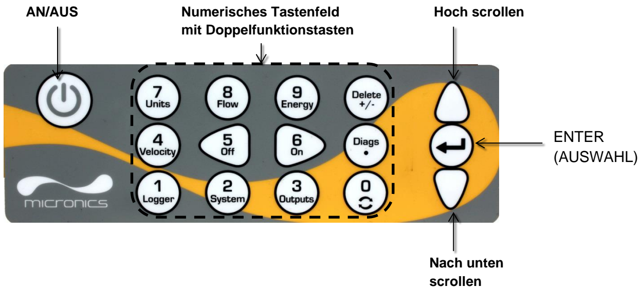
Abbildung 6 Portaflow-Tastenfeld
