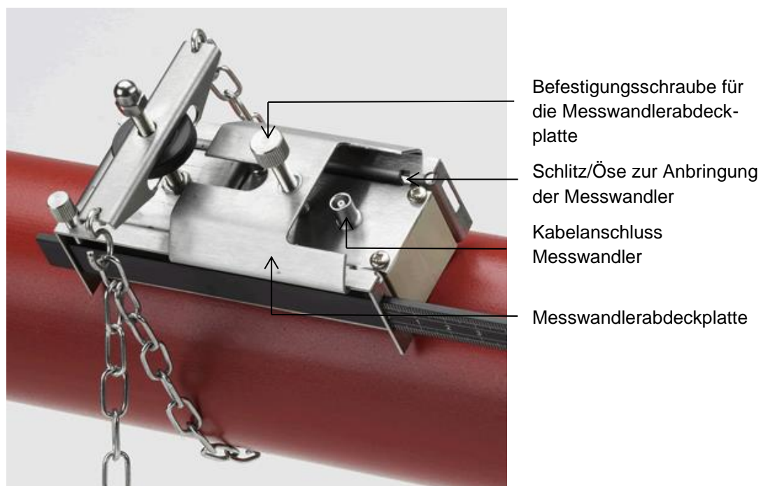
Abbildung 11 Messwandler in der Führungsschiene
