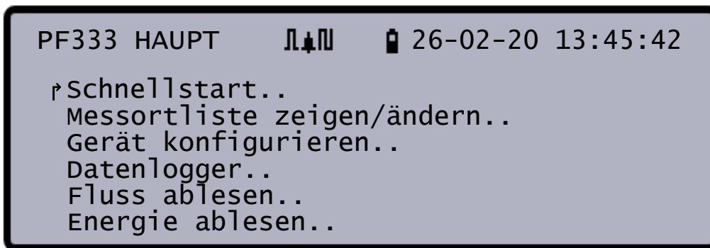
Abbildung 7 Hauptmenü (Optionen Energie ablesen und Datenerfassung nur bei PF333HM-Modellen verfügbar)
