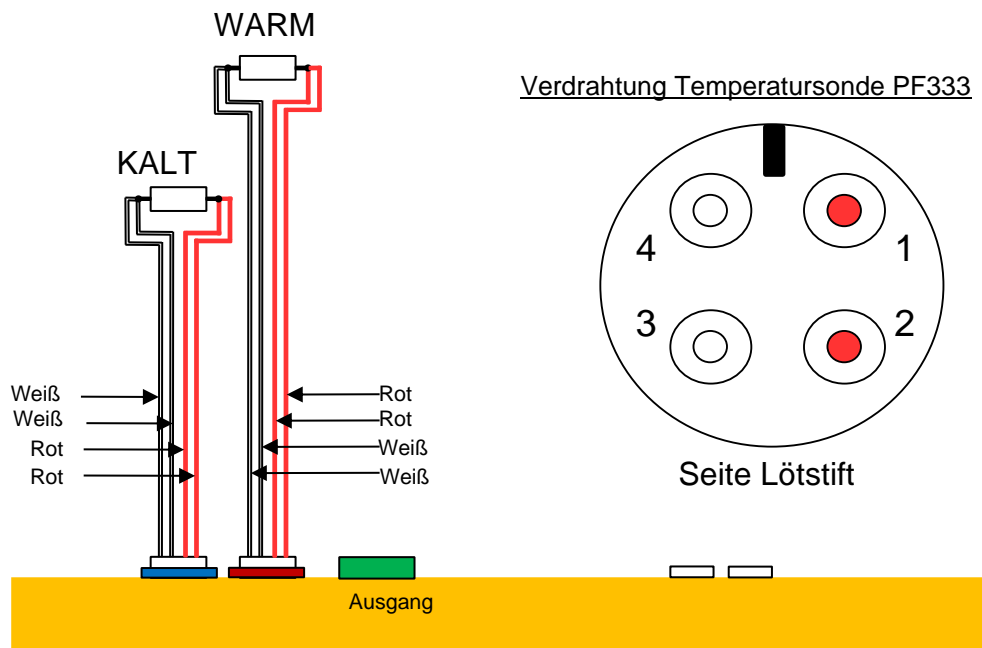
Abbildung 14 Verdrahtung Temperatursonde PF333
