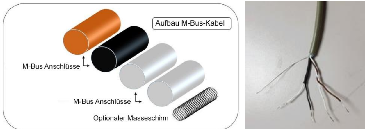
Abbildung 11 Aufbau M-Bus-Kabel
