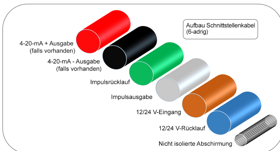
Abbildung 6 6-adriges Hauptschnittstellenkabel
