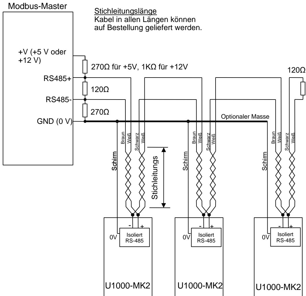
Abbildung 9 Modbus-Anschlussplan
