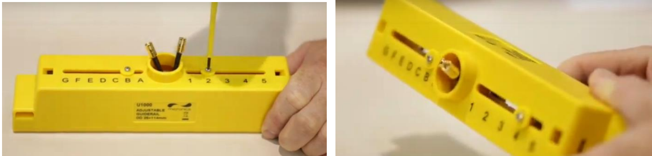
Abbildung 14 Lösen Sie die Schrauben der Durchflusssensorhalterung (links); schieben Sie sie an die richtige Position (rechts)
