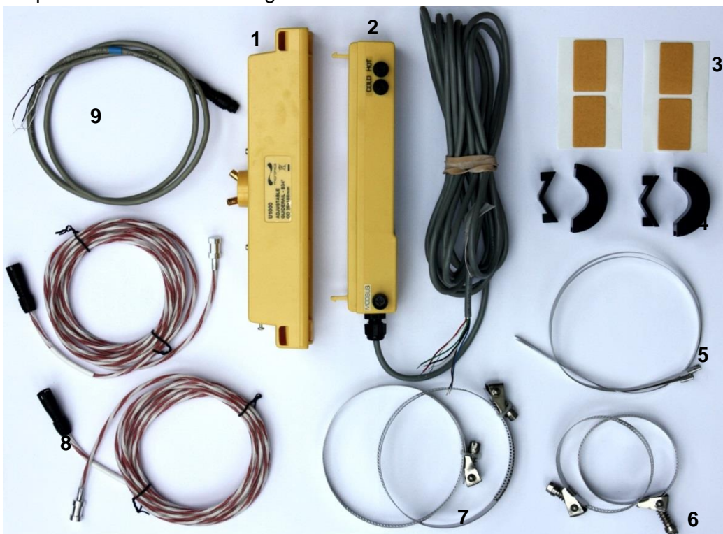
Abbildung 2 Packungsinhalt
