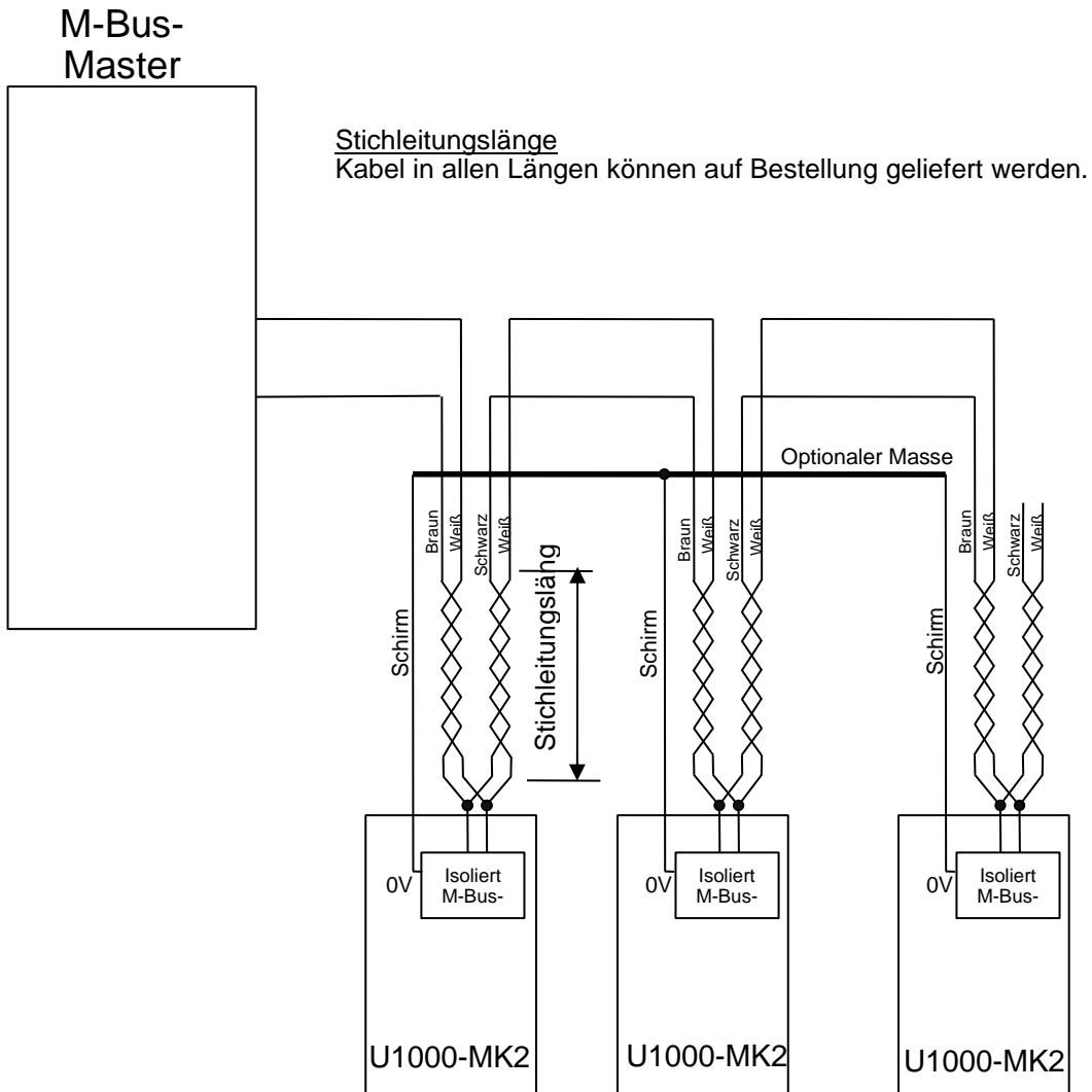
Abbildung 12 M-Bus-Anschlussplan
