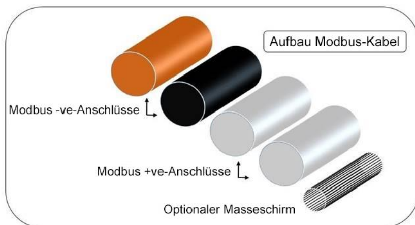
Abbildung 8 Aufbau Modbus-Kabel
